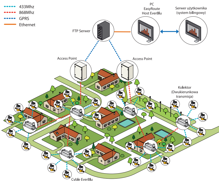
Schemat systemu EverBlu.
